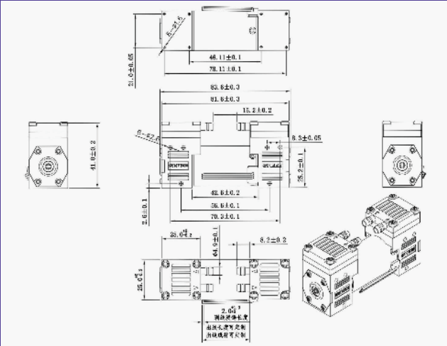
尺寸图 \ Dimension drawing
